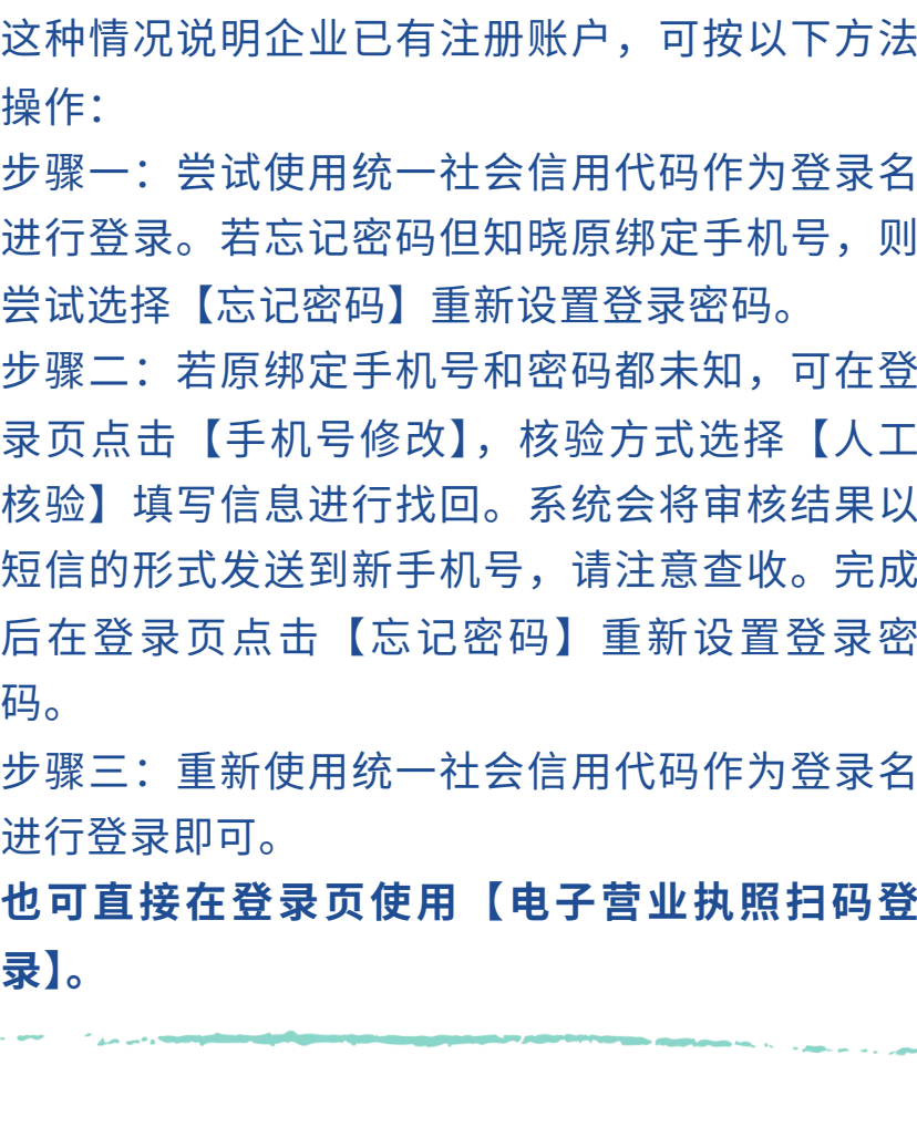
图2 | 用户注册
